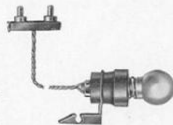
13545 1.30 Schlußlaterne mit roter Glühbirne 13528, Zwerggewinde 9 mm Kabel mit Stecker 13484 S
