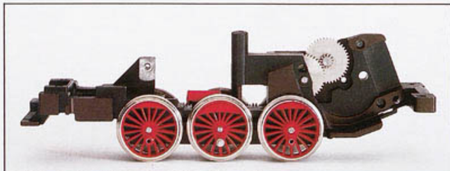
Das Fahrgestell aus Zinkdruckguß ist wartungsfrei.
