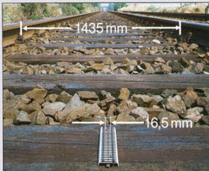
Die Spurweite entspricht maßstabsgetreu der Regelspur der Deutschen Bundesbahn sowie der meisten europäischen Bahnen.
