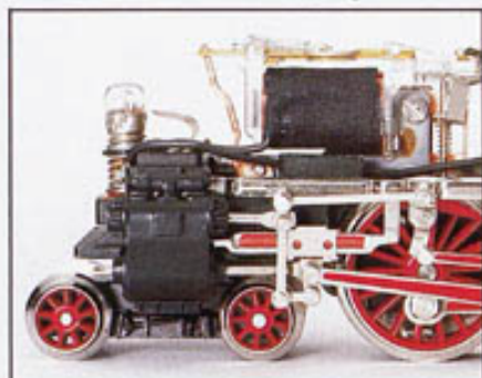
Heusinger Steuerung: Nach dem Eisenbahn-Ingenieur Edmund Waldegg von Heusinger 1817-1886
