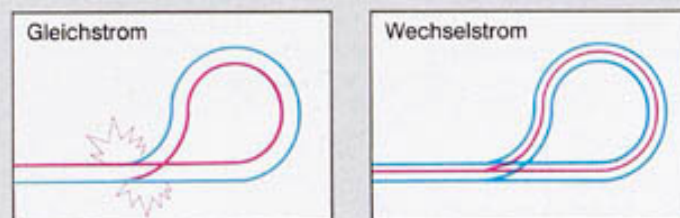
Der Einsatz von Wechselstrom und das Mittelleiter-System ermöglichen einen störungsfreien Stromkreislauf.
