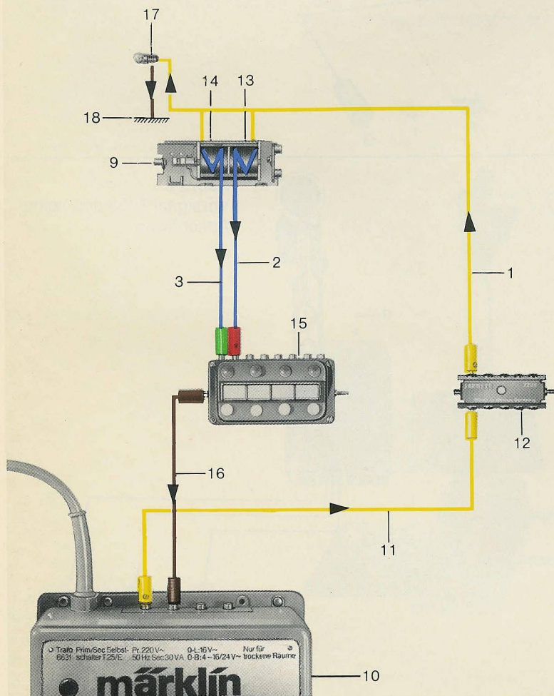
Abb. 3 Verlauf des Signalstell- und Beleuchtungsstromes bei Verwendung der Gleisstücke 5100 und 5200
