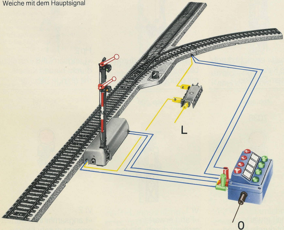
Abb. 20 Gleichzeitige Steuerung einer Weiche mit dem Hauptsignal
