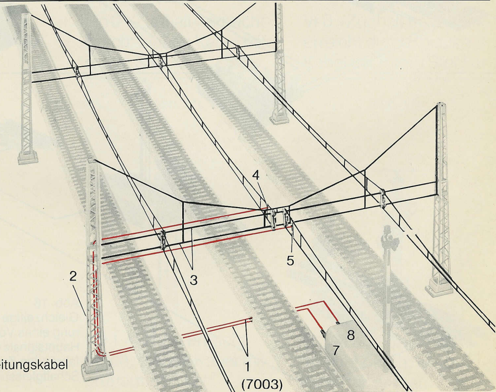
Abb. 13 Oberleitungsstromunterbrechung durch zwei nebeneinander- liegende Fahrdrahtisulierungen 7006
