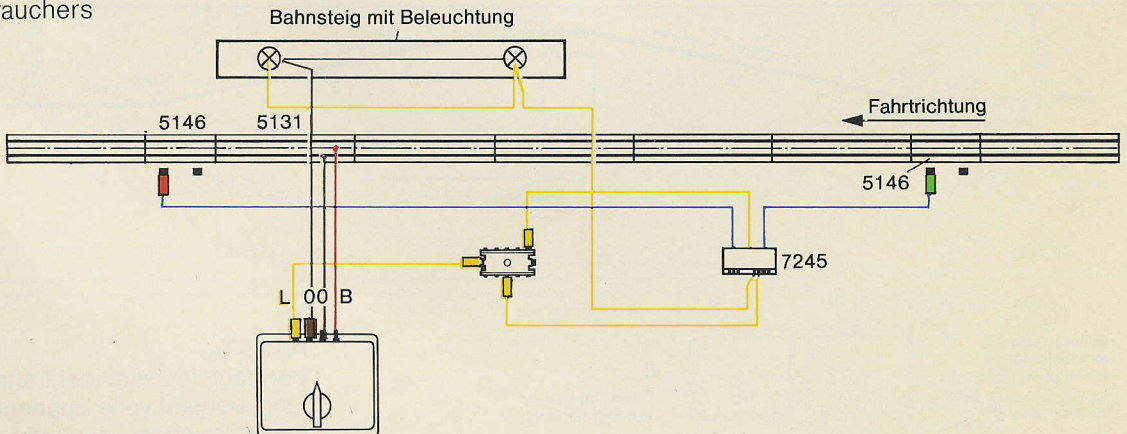
Abb. 38 Ein- und Ausschalten eines Verbrauchers
