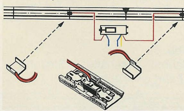
Abb. 11 Anbringen der Kontaktlaschen
