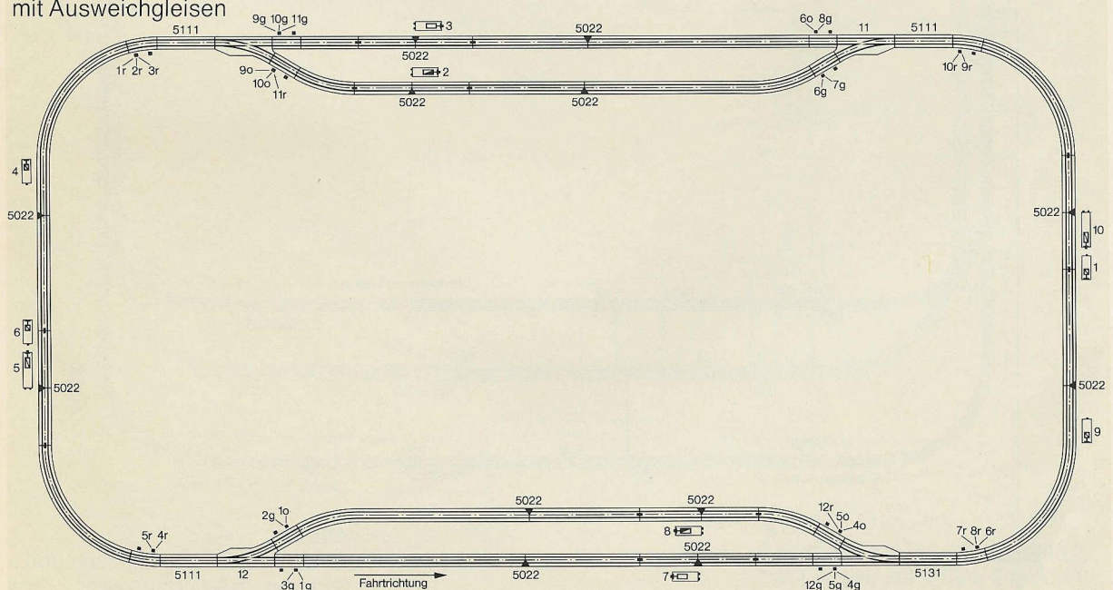
Abb. 33 Blockbetrieb auf einer Anlage mit Ausweichgleisen
