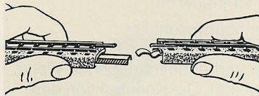
Abb. 10 Anbringen der Mittelleiter- isolation 5022
