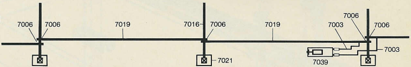
Abb. 13 Oberleitungsstromunterbrechung durch zwei nebeneinander- liegende Fahrdrahtisulierungen 7006
