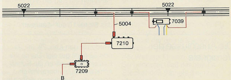
Abb. 35 Schaltung bei Stromzuführung über das Schaltpult 7210
