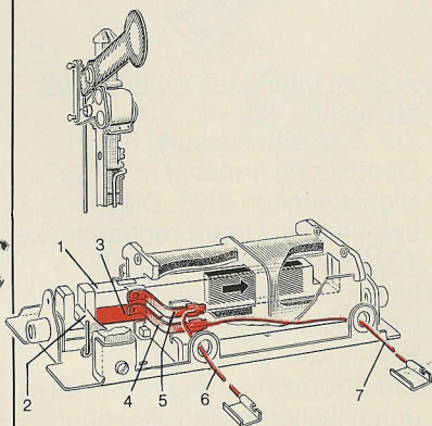
Abb. 8a Bahnstromschalter in Stellung »Fahrt«
