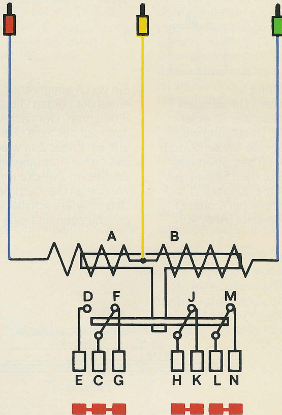
Abb. 37 Die elektrische Funktion des Universalferschalzers
