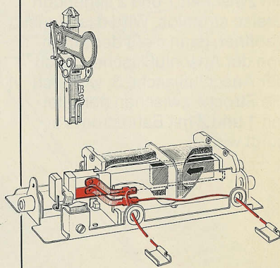
Abb. 8b Bahnstromschalter in Stellung »Zughalt«
